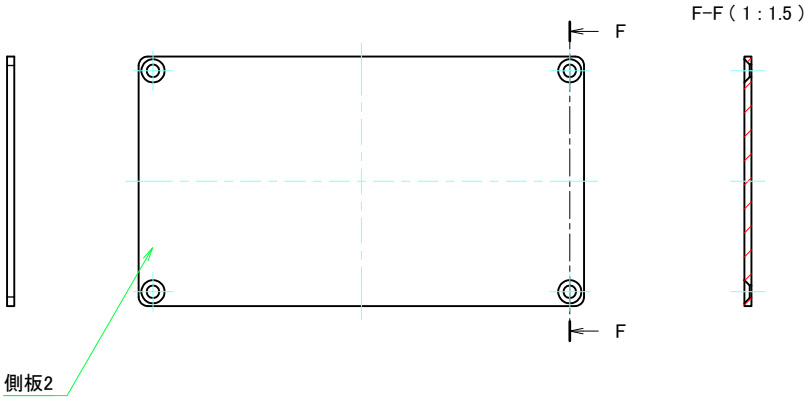
F-F ( 1 : 1.5 )
