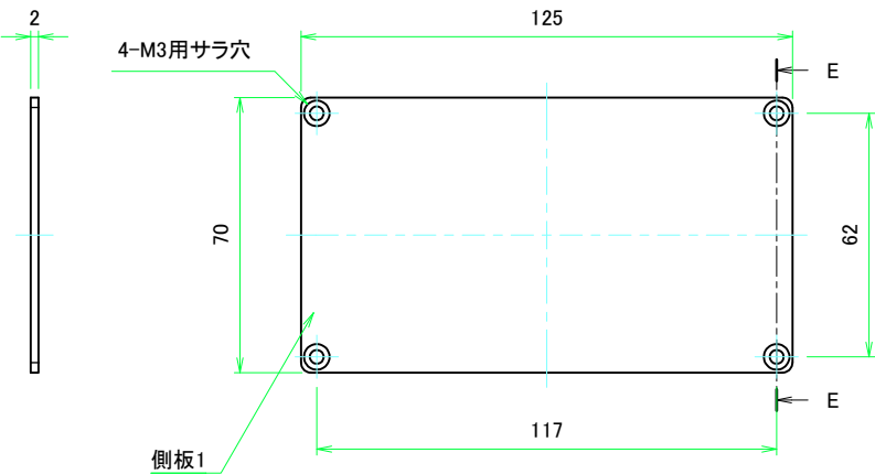
E-E ( 1 : 1.5 )
