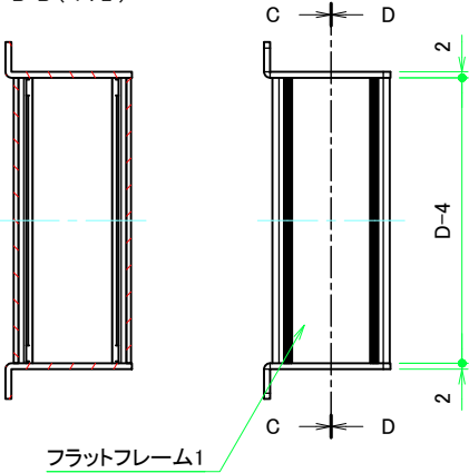
B-B (1:2)
