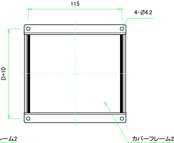
D-D (1:2)
