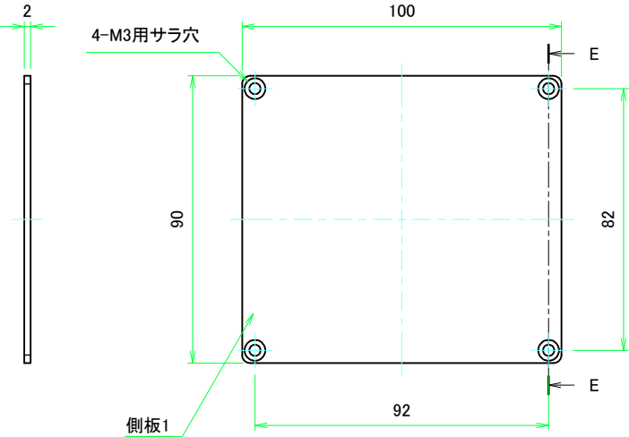
E-E ( 1 : 1.5 )
