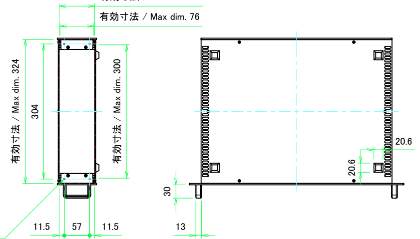
A-A (1:6)
