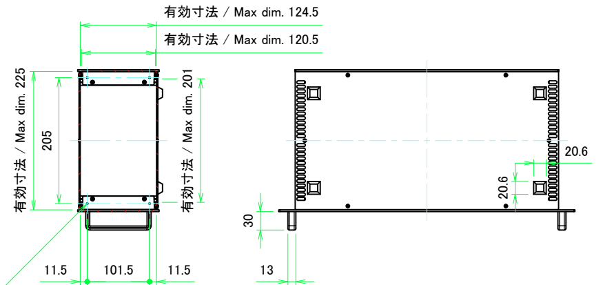
A-A (1:6)
