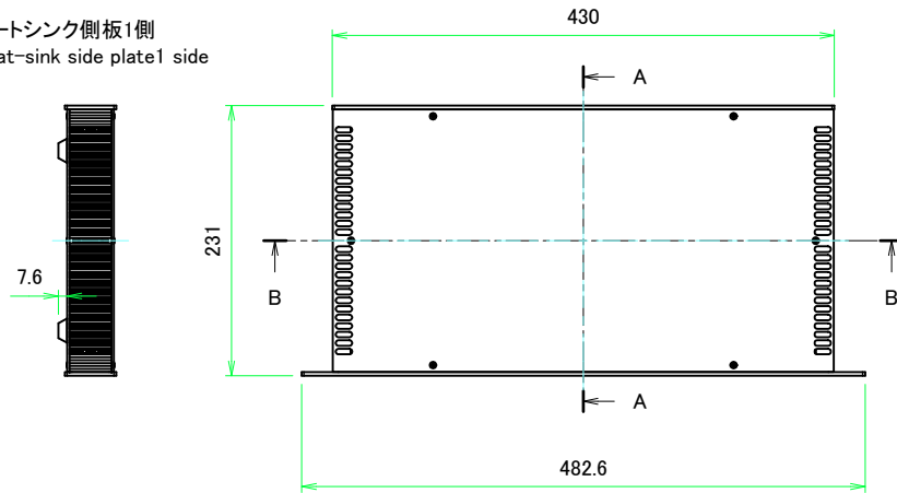
ヒートシンク側板2側 Heat-sink side plate2 side
