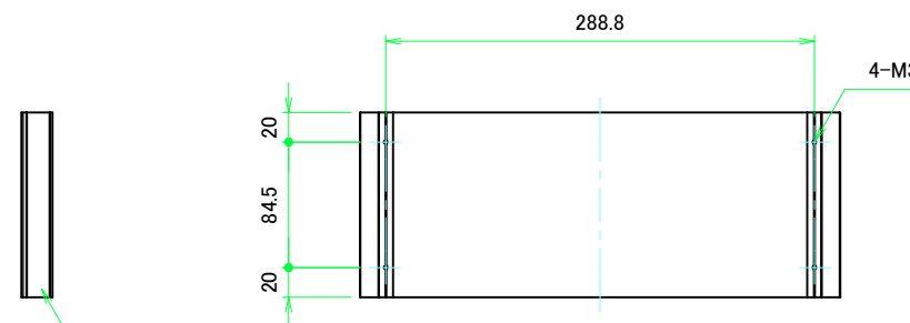
ヒートシンク側板1 / Heat-sink side plate1
