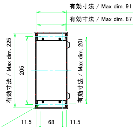
A-A (1:5)
