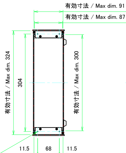
A-A (1:5)
