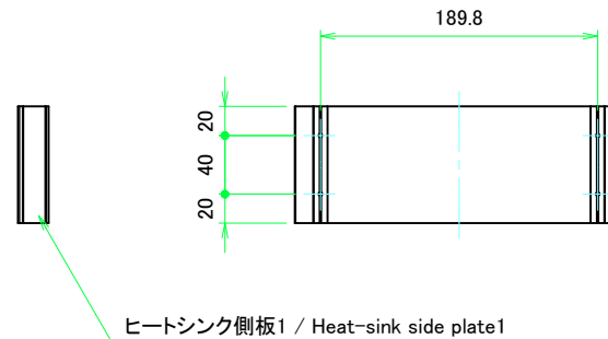
ヒートシンク側板1 / Heat-sink side plate1
