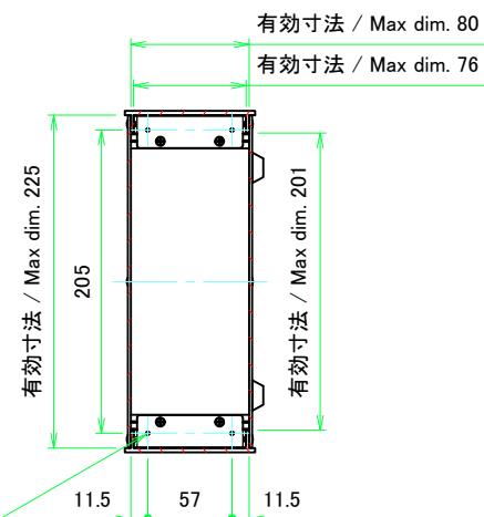
A-A (1:4)
