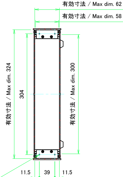
A-A (1:4)
