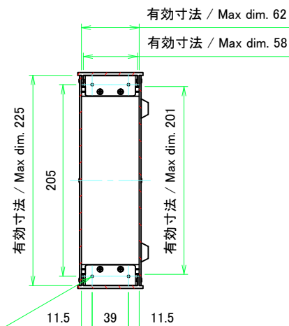
A-A (1:4)
