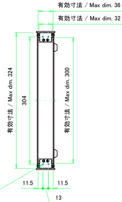
A-A (1:4)
