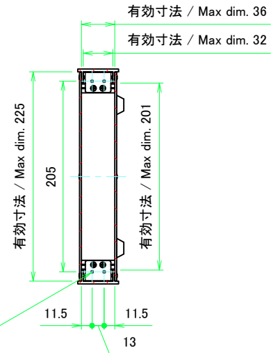
A-A (1:4)
