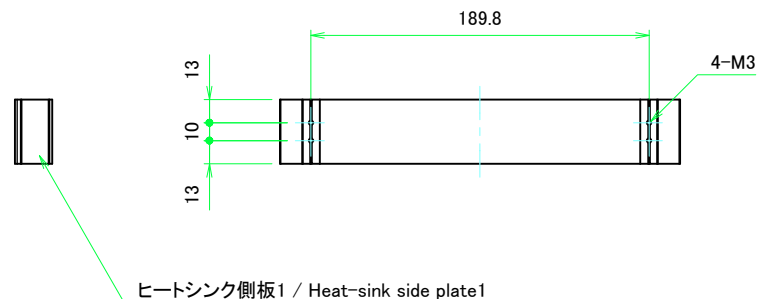
ヒートシンク側板1 / Heat-sink side plate1
