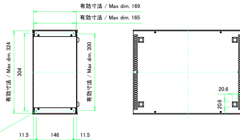
A-A (1:6)
