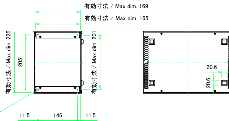
A-A (1:6)
