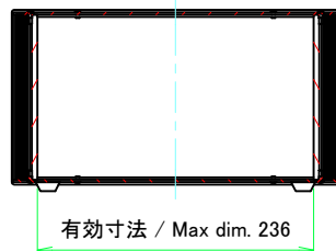
B-B ( 1 : 5 )
