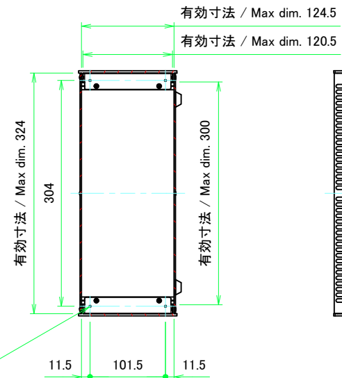
A-A (1:5)
