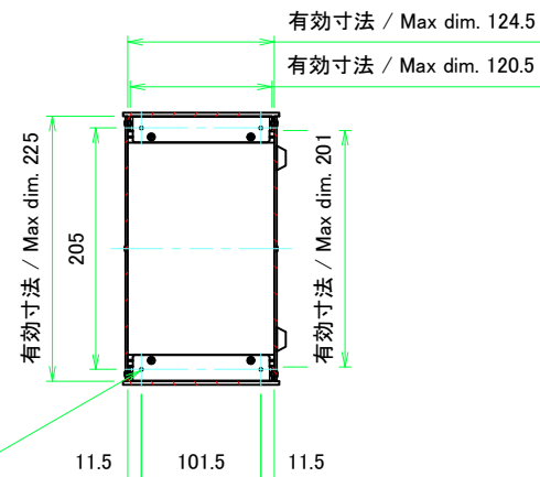
A-A (1:5)
