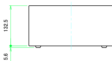
B-B ( 1:5 )
