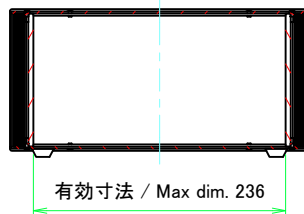
B-B ( 1:5 )
