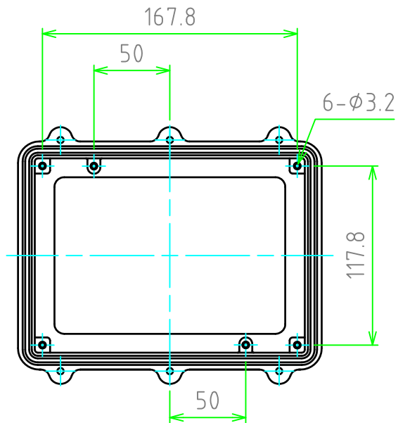
トップカバー（内視）
