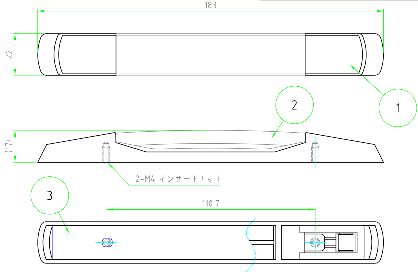
取付穴寸法図
