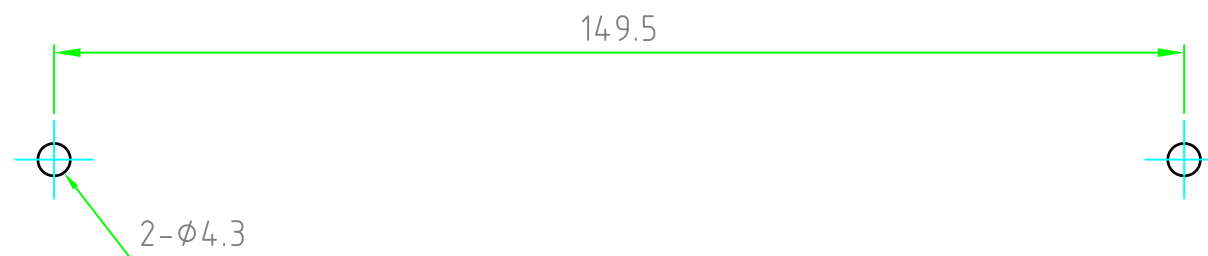
取付穴寸法図
