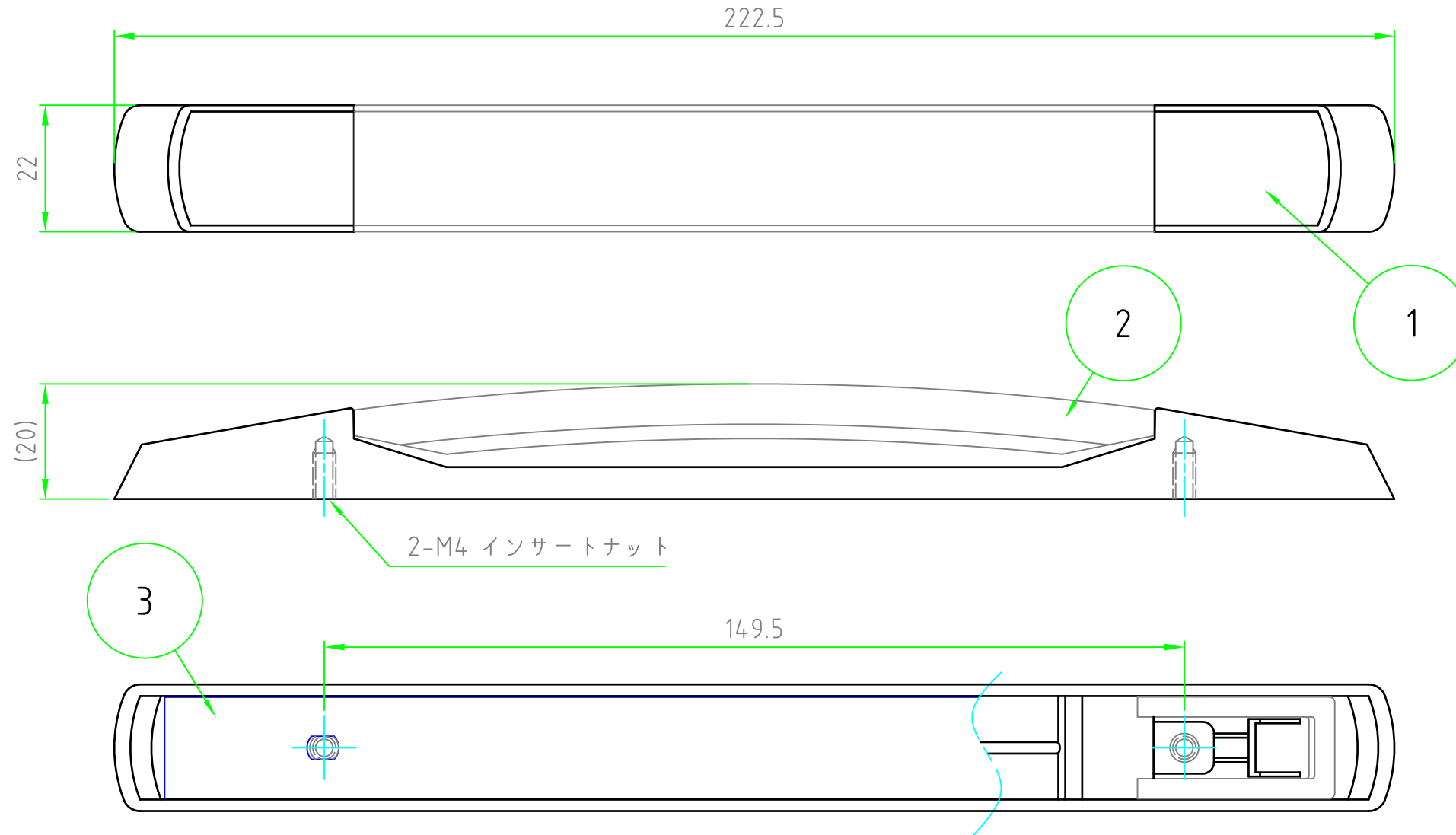
取付穴寸法図
