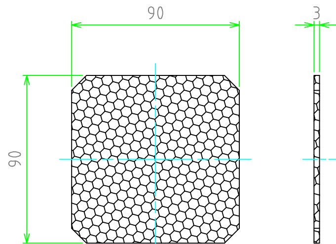
フィルター寸法図
