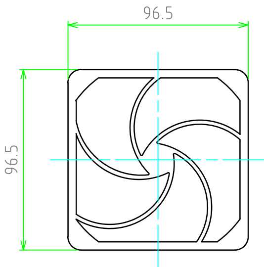
はめ込みカバー寸法図
