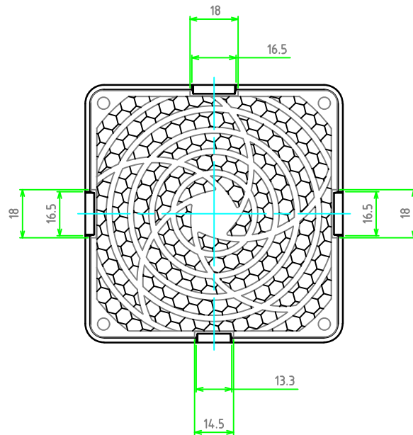
取付カバー寸法図
