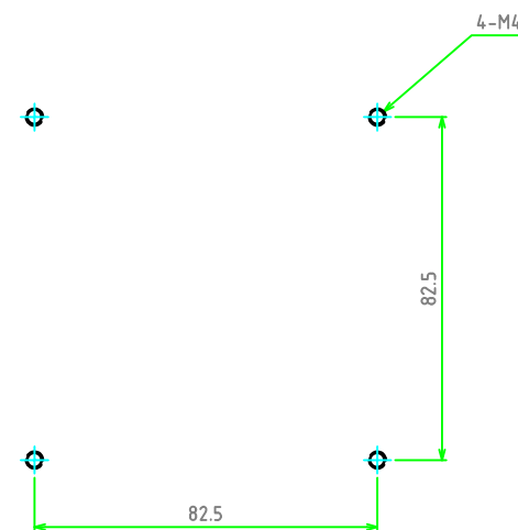
取付穴寸法
