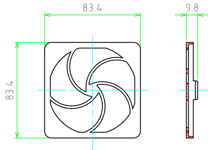
はめ込みカバー寸法図
