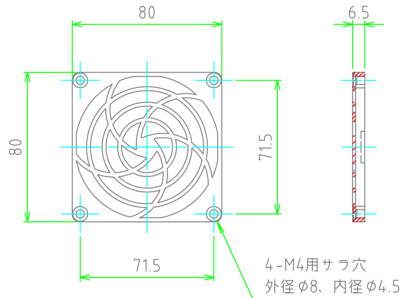
取付カバー寸法図
