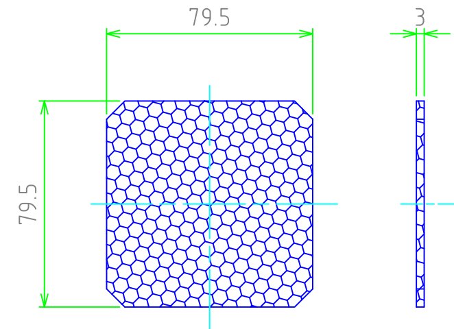
フィルター寸法図
