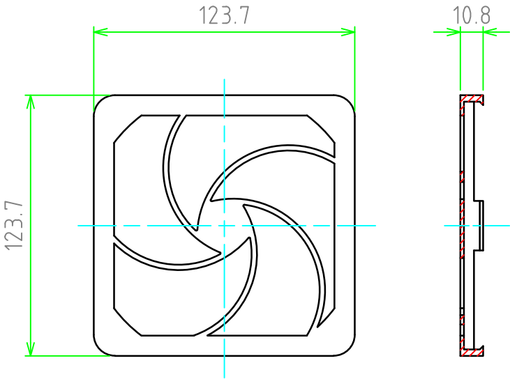
はめ込みカバー寸法図
