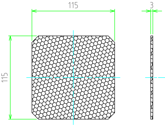
フィルター寸法図
