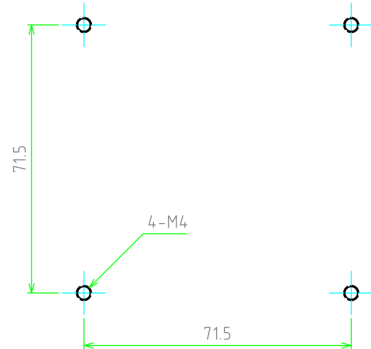
取付穴寸法
