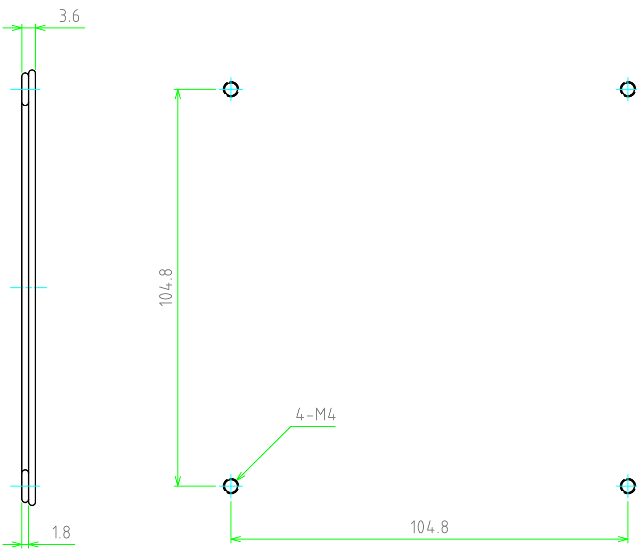
取付穴寸法
