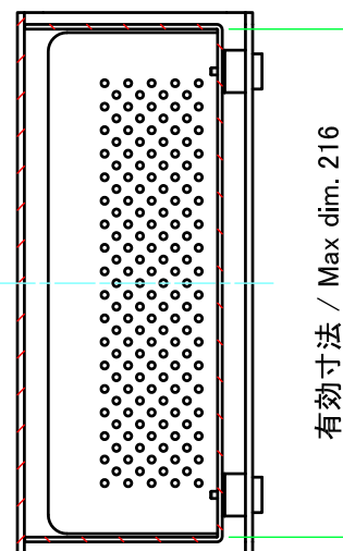
B-B ( 1:3.5 )
