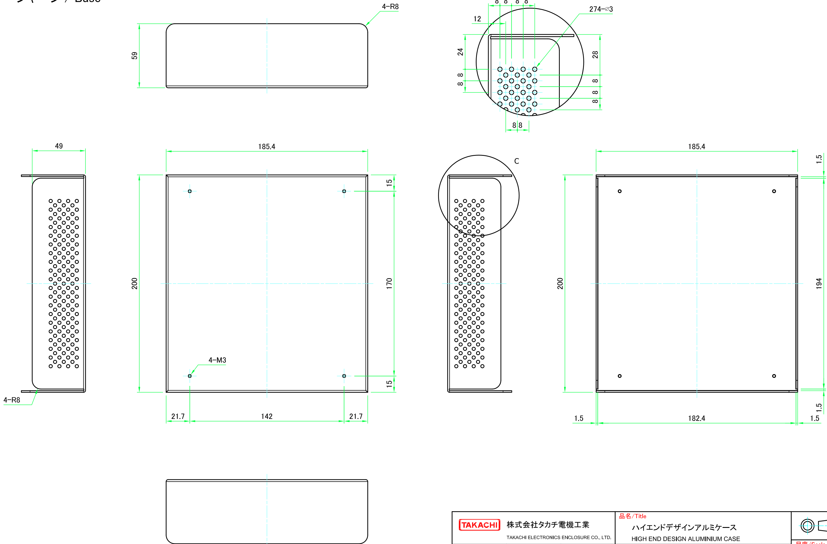
C : 放熱穴 拡大図 Ventilation holes
