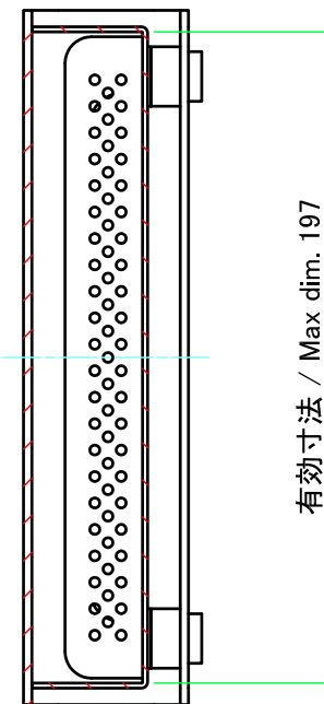
B-B ( 1 : 2.5 )
