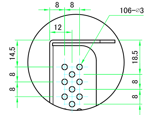
C : 放熱穴 拡大図
