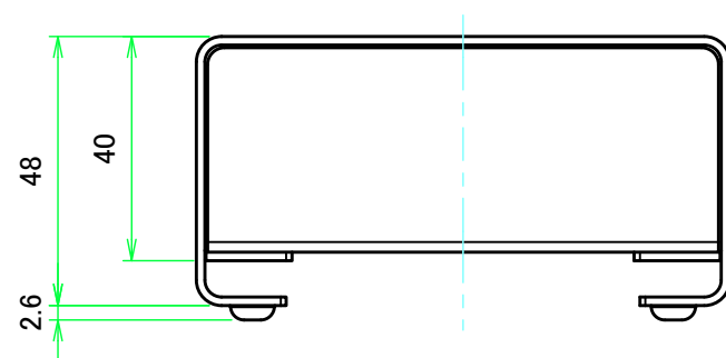
A-A ( 1 : 1.5 )
