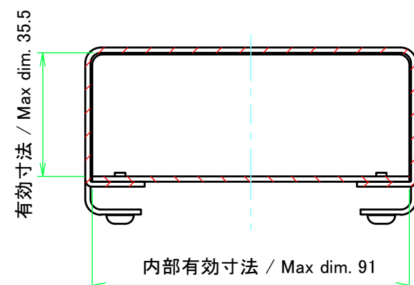
A-A ( 1 : 1.5 )
