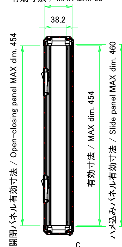
B-B (1 : 6)
