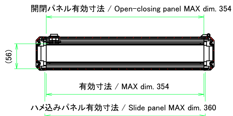
A-A (1:5)
