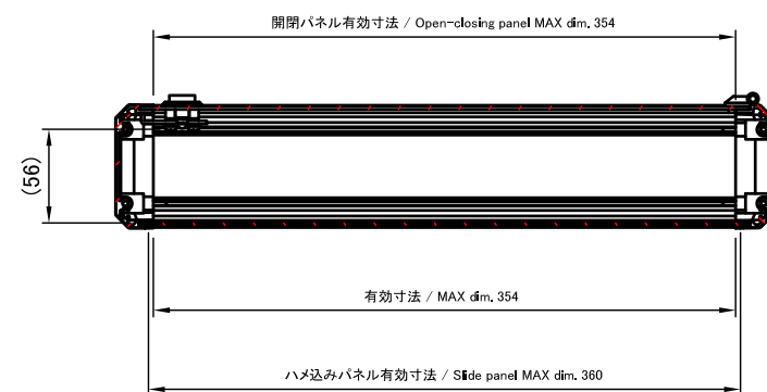
A-A ( 1 : 5 )
