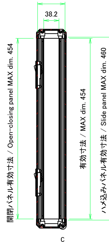
有効寸法 / MAX dim. 69
