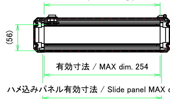
開閉パネル有効寸法 / Open-closing panel MAX dim. 254
