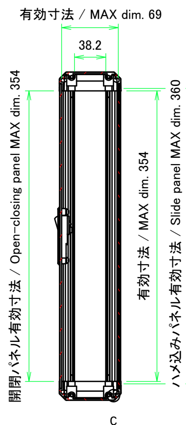
B-B ( 1 : 4.5 )
