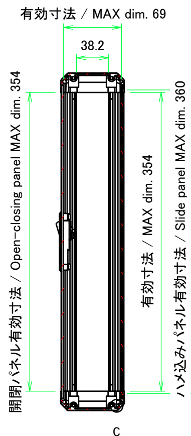
B-B ( 1 : 4.5 )
