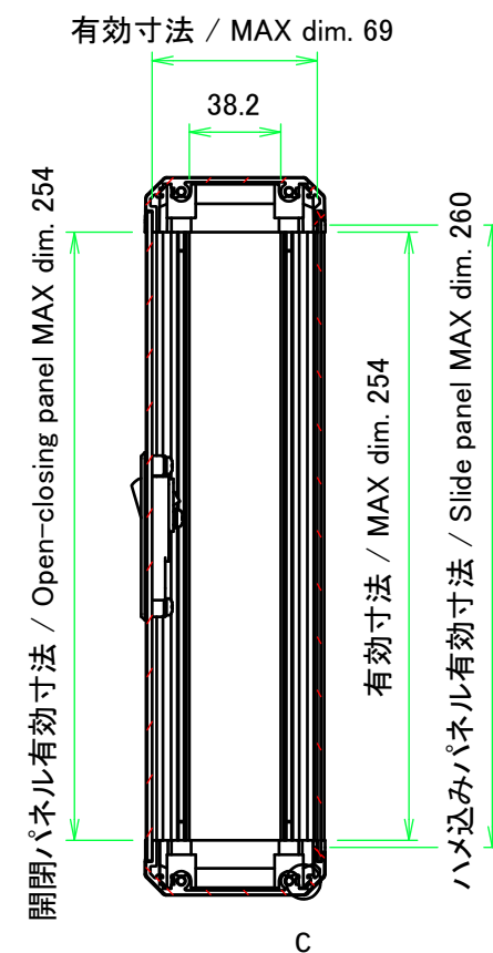
B-B ( 1 : 3.5 )
