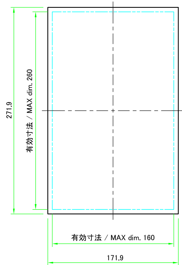
パネル表面 / Panel Frontside
