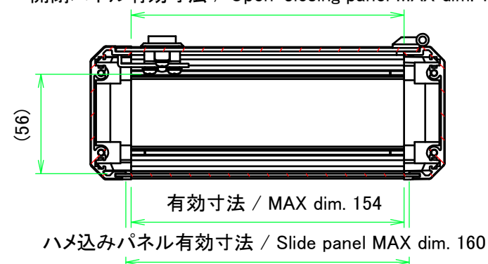
A-A (1:3)
