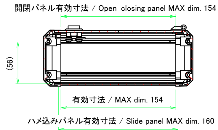
A-A (1:3)
