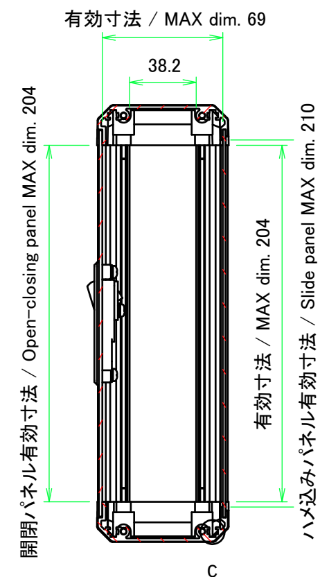
B-B ( 1 : 3 )
