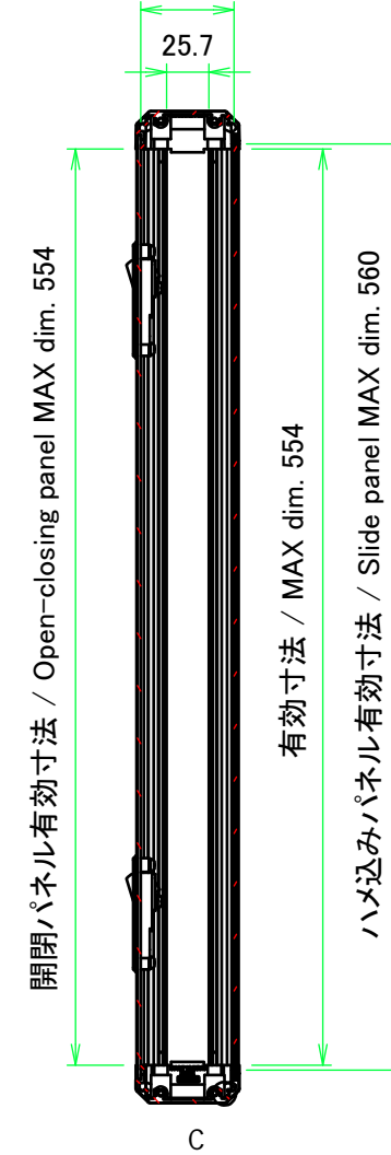
C: フレーム拡大図 / Frame cross-section
