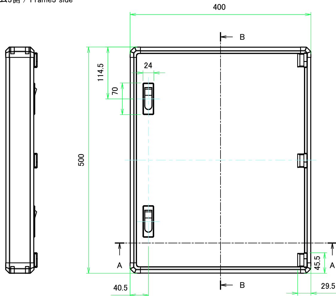
フレーム3側 / Frame3 side
