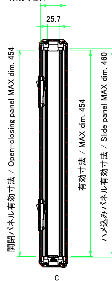
C: フレーム拡大図 / Frame cross-section
