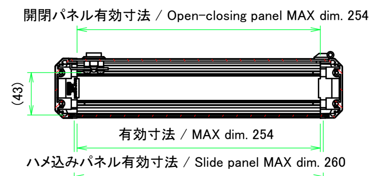
A-A (1:4)
