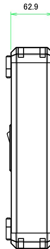
フレーム4側 / Frame4 side
