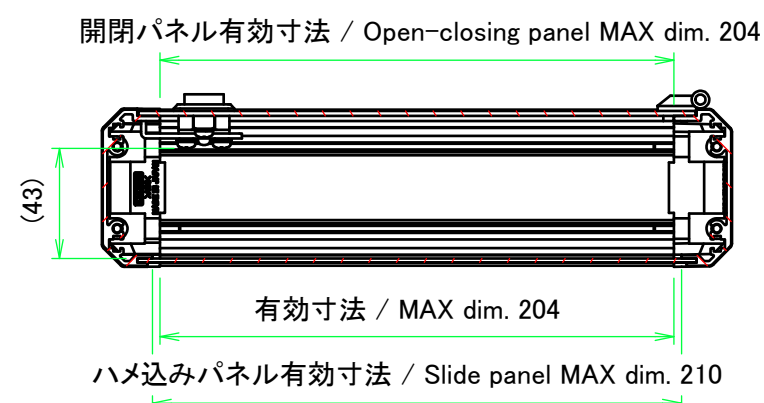
A-A (1:3)
